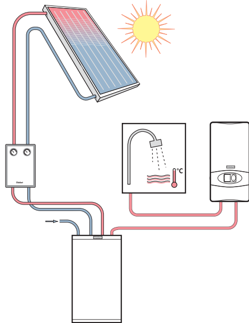
VED E model cihazın auroSTEP 150 paket solar sistem bağlantılı akım şeması
